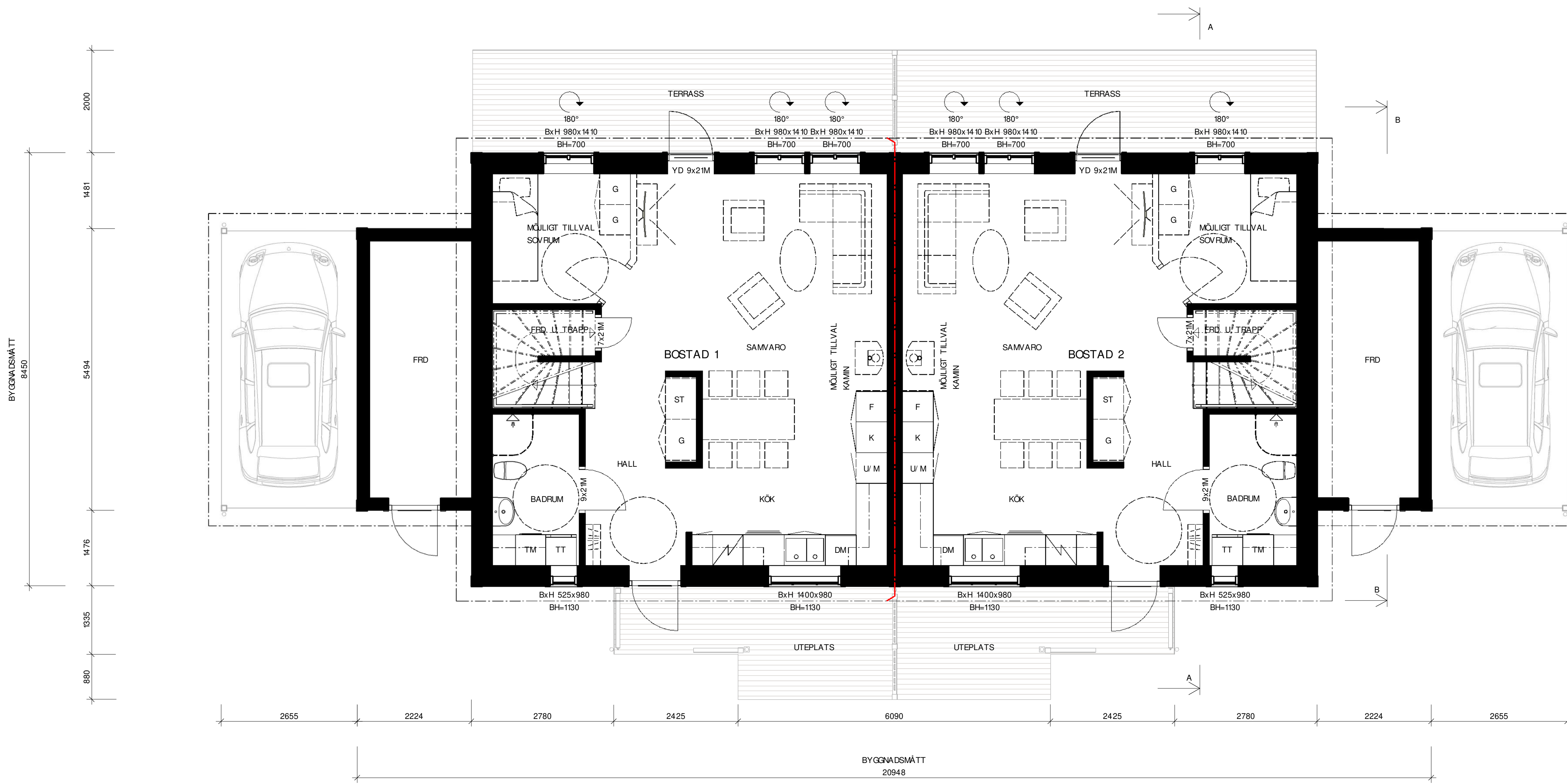
BOTTENVÅNING SKALA 1:50
