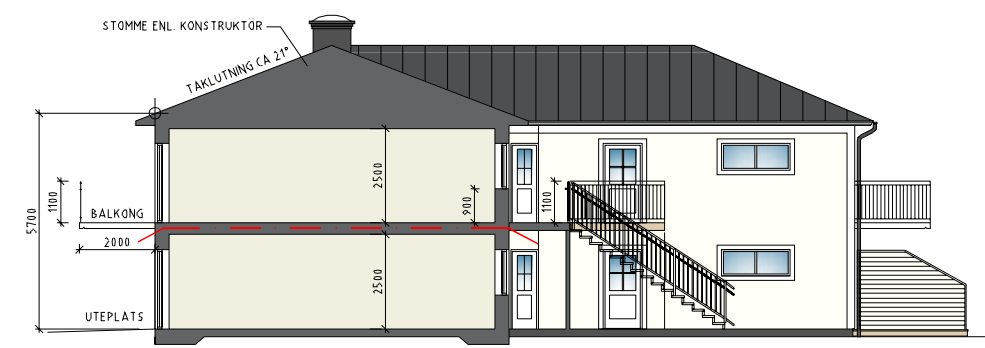
INNERFASAD MOT NORR & PRINCIPSEKTION
